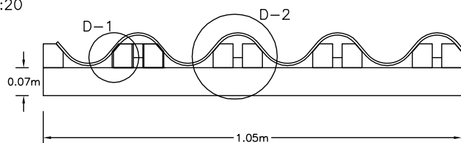
ALZADO FRONTAL ESCALA 1:10
