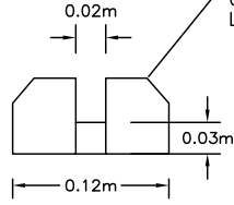
DETALLE 2 ESCALA 1:5
