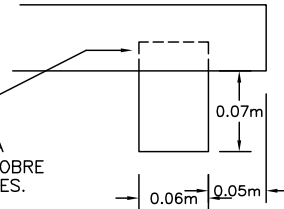
DETALLE 3 ESCALA 1:5
