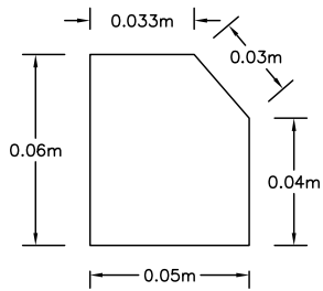
DETALLE 1 ESCALA 1:2
