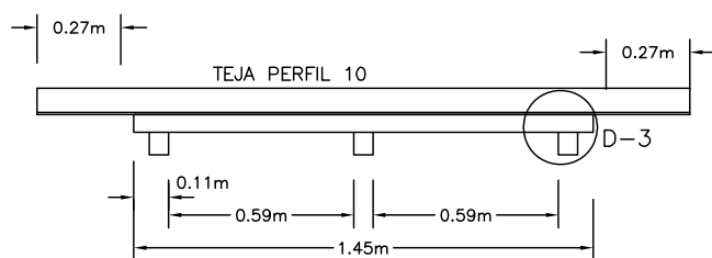
ALZADOS LATERALES ESCALA 1:20
